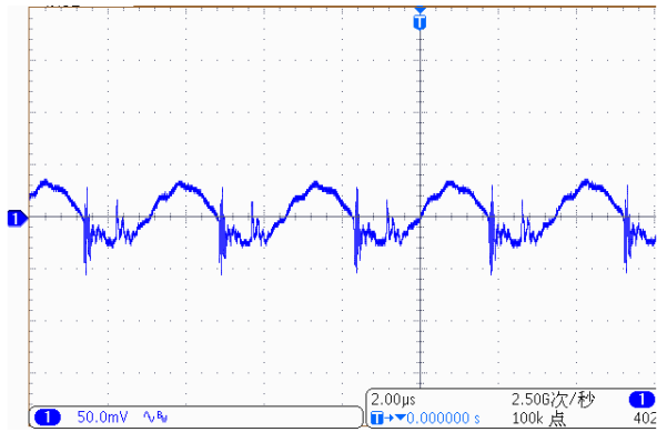
V_{in}=110Vdc, I_o=12.5A (20MHz)
