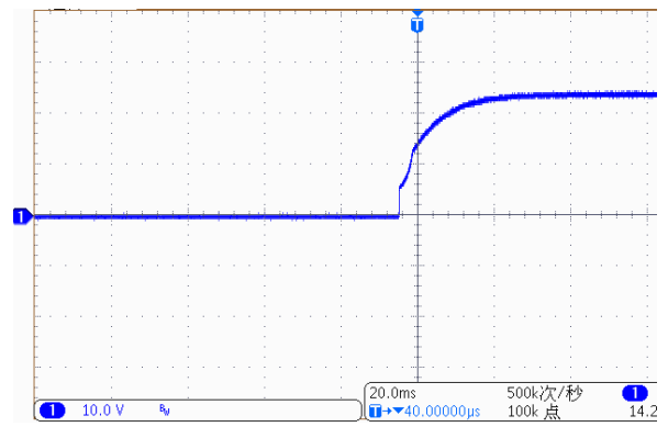
V_{in}=110Vdc, I_o=12.5A (20MHz)
